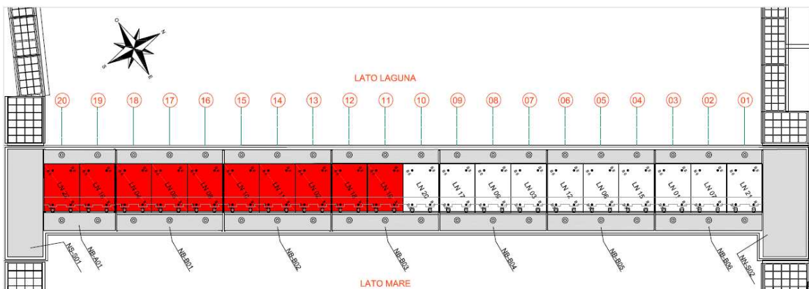
FIG. 1 - PARATOIE OGGETTO DI SOLLEVAMENTO GIORNATA 5
